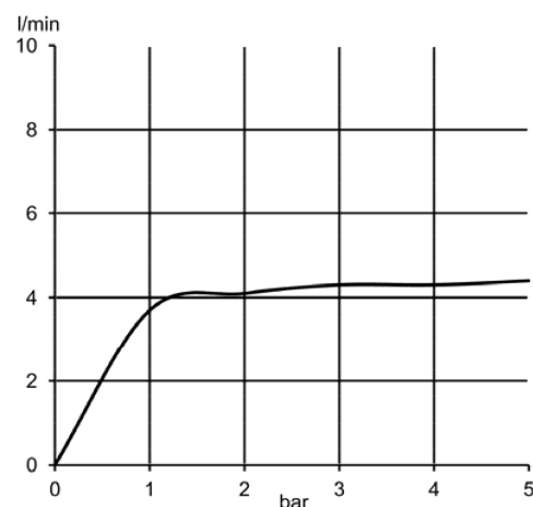
Diagram przepływu
