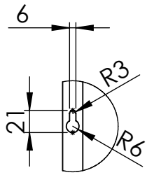
SZCZEGÓŁ A SKALA 1 : 5
