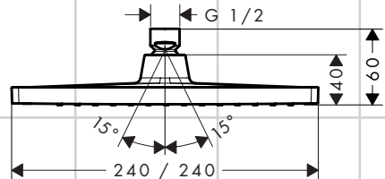
Crometta E 240 1jet 26726000
